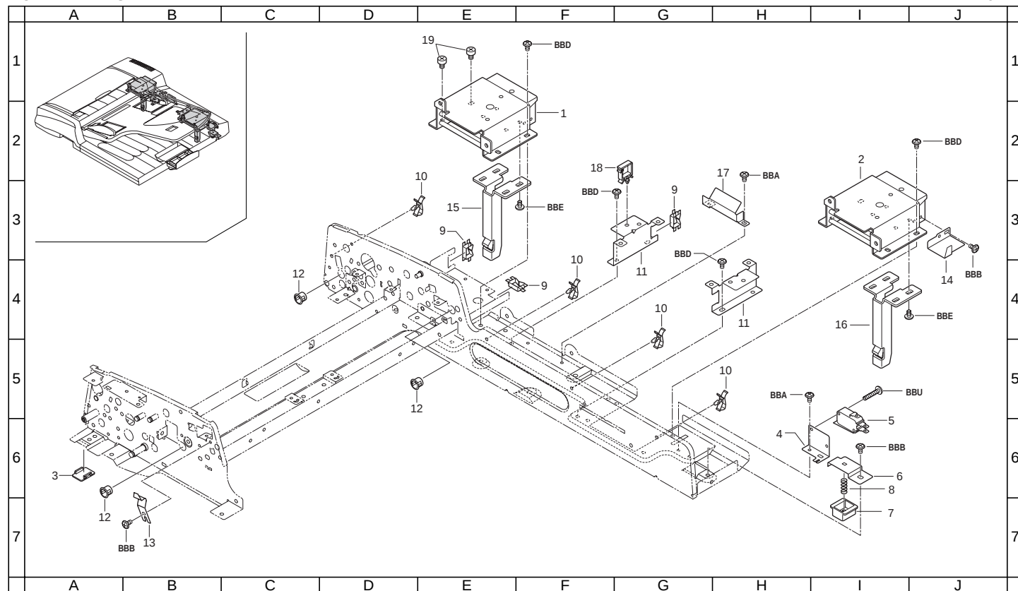
FIG. 2 FRAMES
