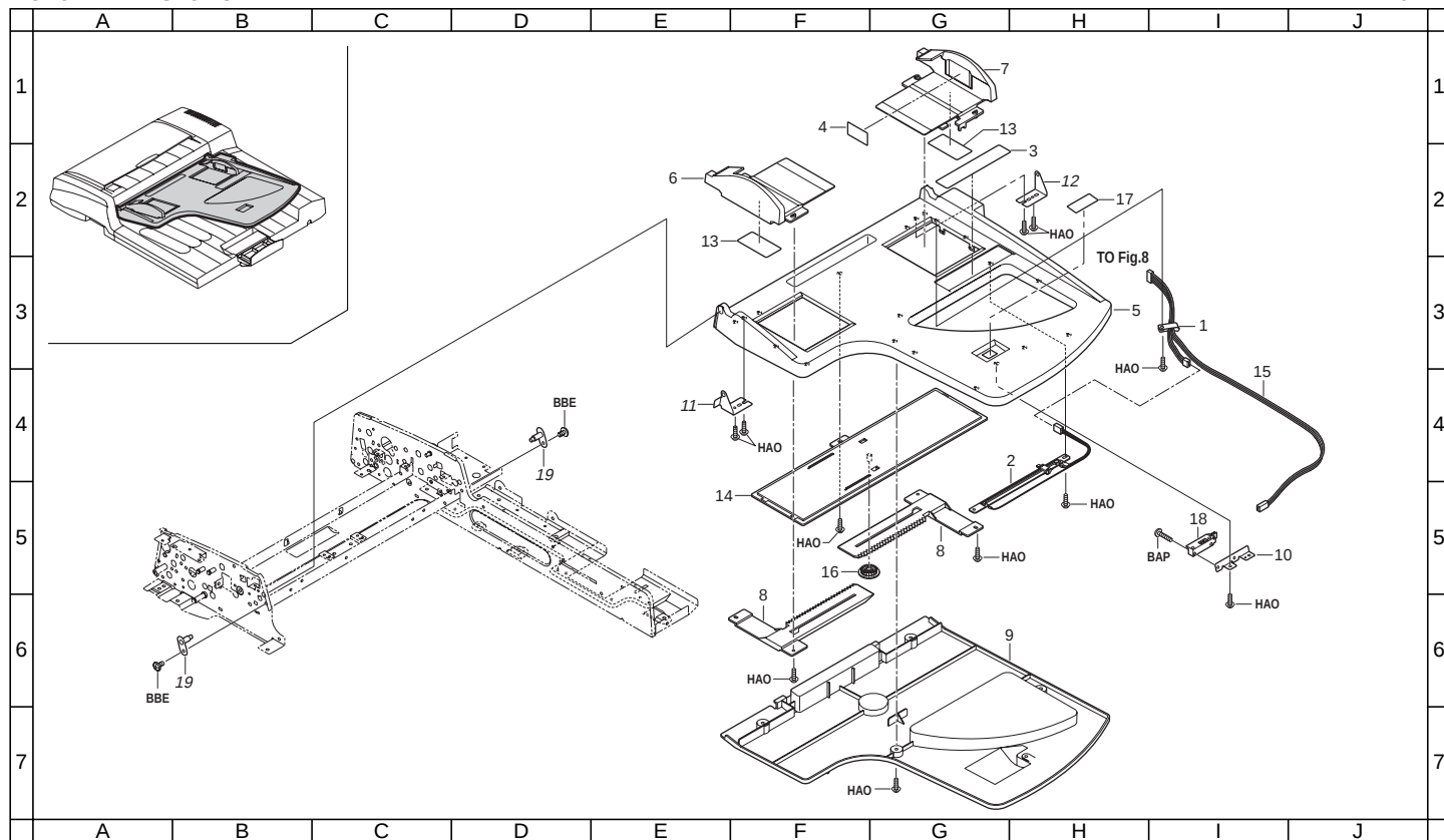
FIG. 3 TABLE SECTION
